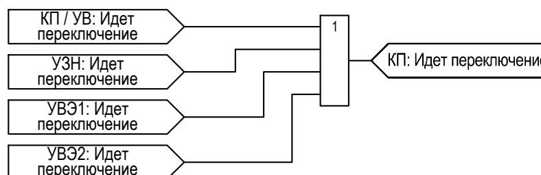
Рисунок 2.54 – Функциональная схема формирования общего сигнала переключения коммутационного аппарата
